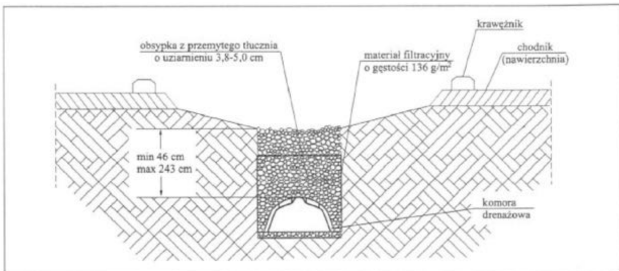
Rys. 2. Mulilo chłonna z komorą drenazową jako elementem retencyjno-filtracyjnym
