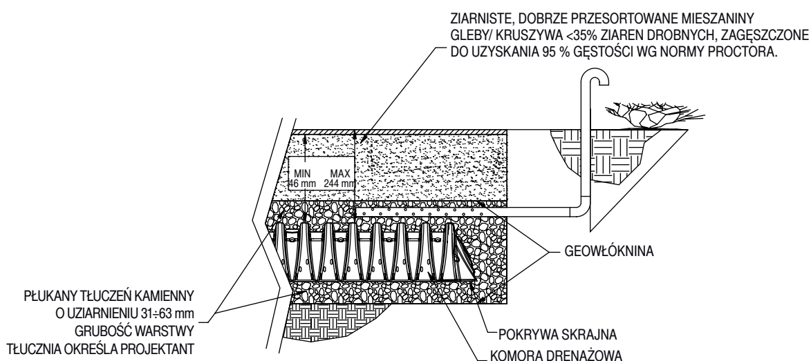
Rys. 15. Odpowietrzenie (rysunek bez zachowania skali)
