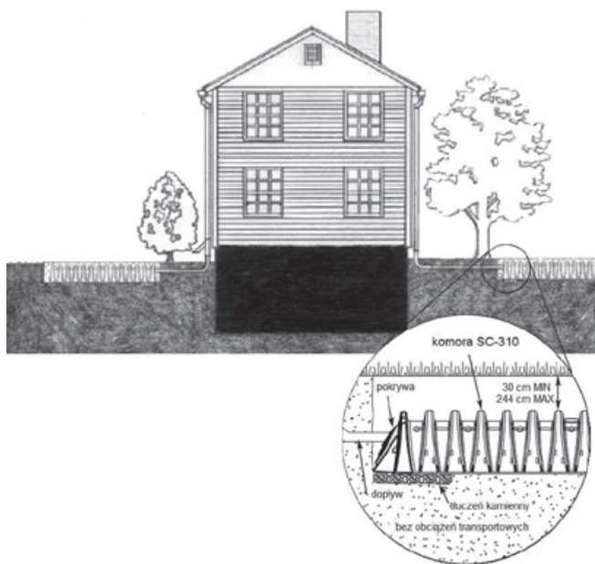
Rys. 10a. Wykorzystanie systemu komór drenażowych SC dla domu jednorodzinnego
