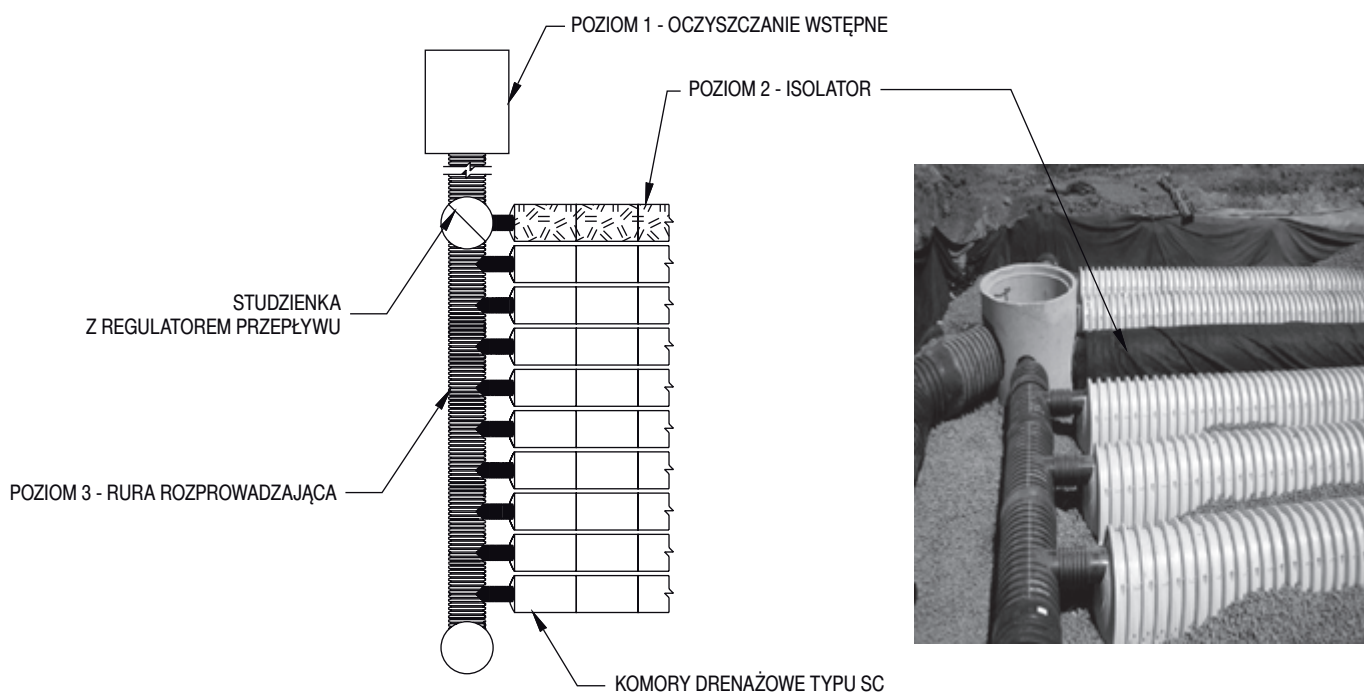
Rys. 1. Izolator zawieszin Isolator™
