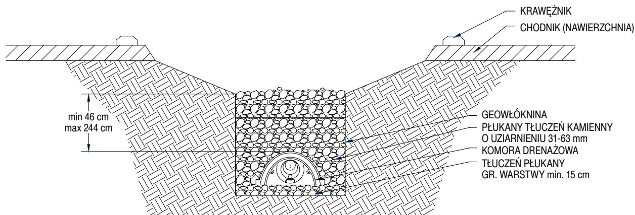
Rys. 16. Zastosowanie systemu komór drenazowych SC jako rów odwadniający.
