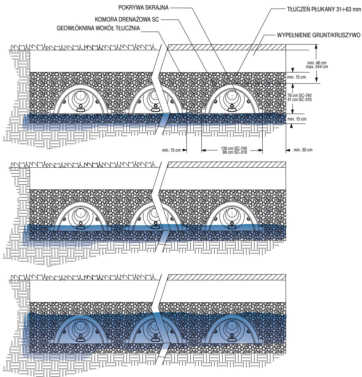
Rys. 8. Etapy wypełniania systemu komór drenazowych SC wodą
