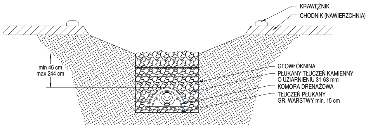
Rys. 10b. Zastosowanie systemu komór drenazowych SC jako rów odwadniający.
