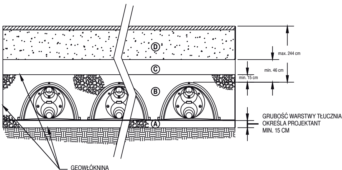
Rys. 11. Rozmieszczenie materiału wypełniającego
