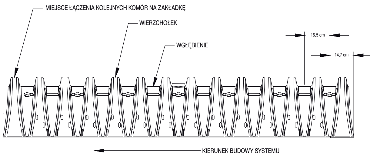
Rys. 5. Komora SC – odległości pomiędzy połaďowaniami
