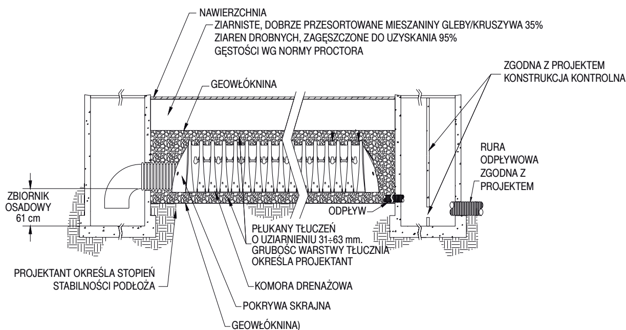
Rys. 14. Rysunek dopływu do komory oraz wylotu z komory (rysunek bez zachowania skali)
